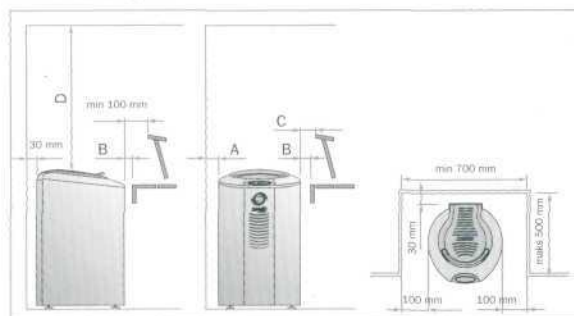
Minimalne odległości
